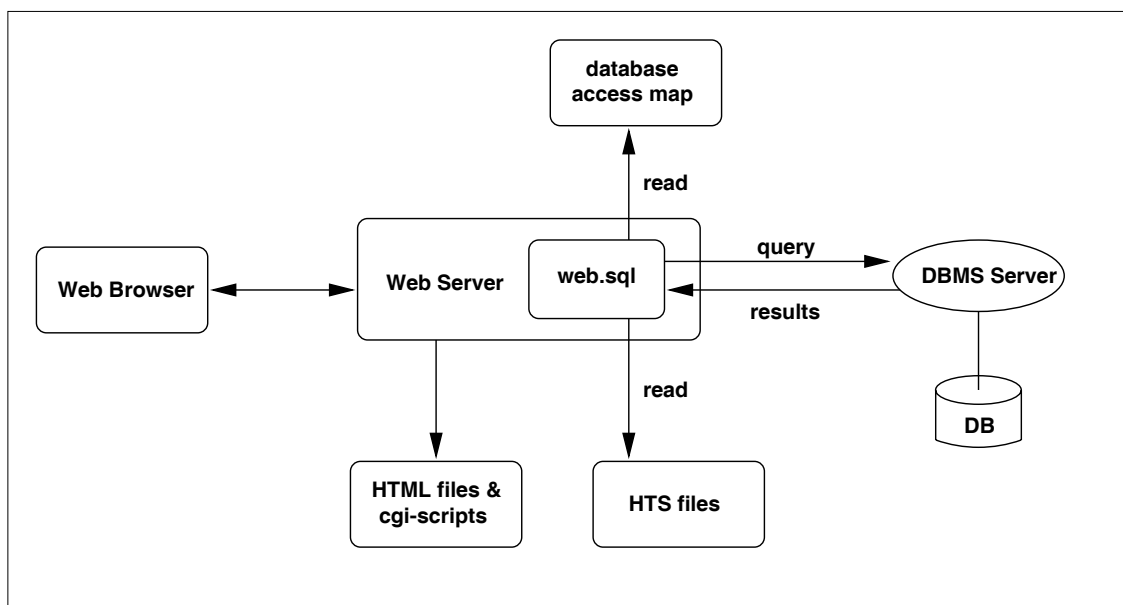
Σχήμα 2.12: Η αρχιτεκτονική που χρησιμοποιεί η Sybase
