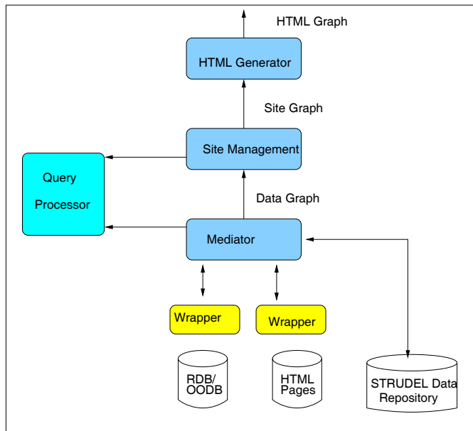
Σχήμα 2.16: Η αρχιτεκτονική του συστήματος Strudel
