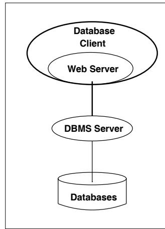
Σχήμα 2.13: Η αρχιτεκτονική Proprietary Server
