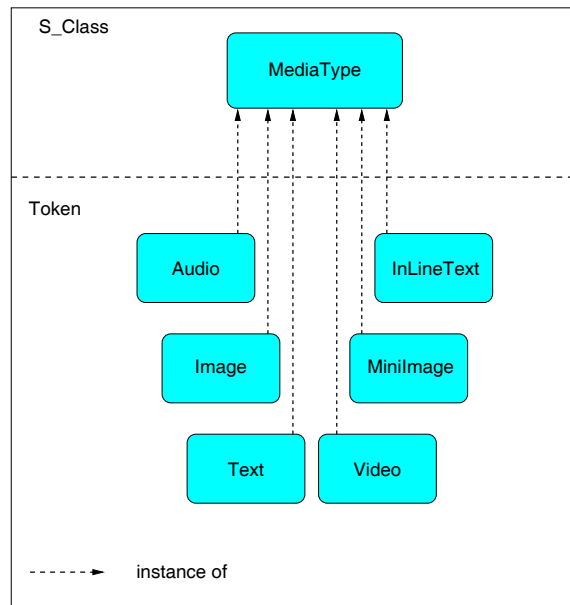
Σχήμα 3.14: Η κλάση MediaType και οι περιπτώσεις της.
