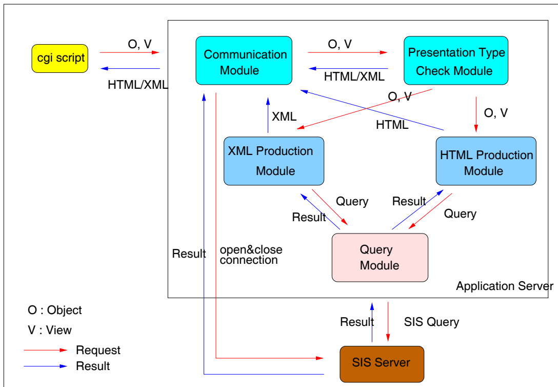
Σχήμα 4.3: Ο εξυπηρετής εφαρμογής υποστηρίζει παρουσίαση σε HTML και XML
