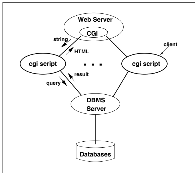
Σχήμα 2.3: Η αρχιτεκτονική CGI executable
