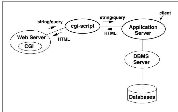
Σχήμα 2.6: Η αρχιτεκτονική CGI Application Server
