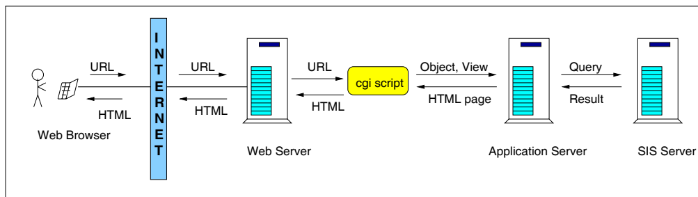
Σχήμα 4.1: Γενική άποψη της αρχιτεκτονικής που υλοποιήθηκε
