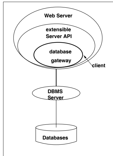
Σχήμα 2.11: Η αρχιτεκτονική Server API
