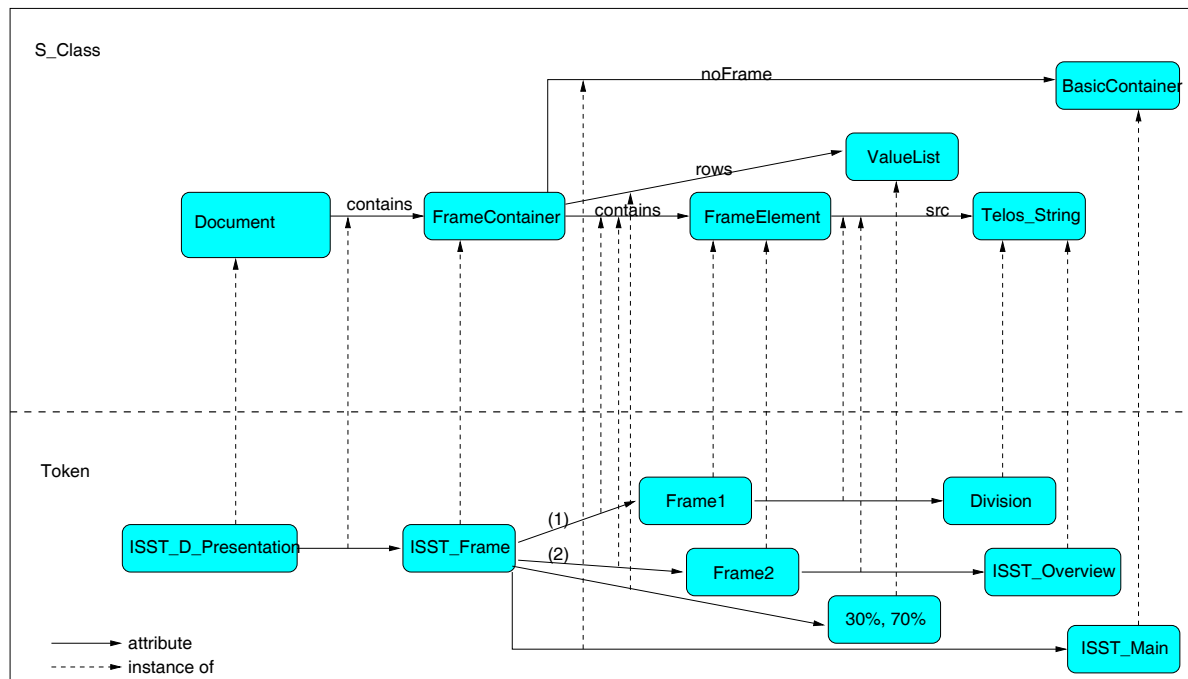
Σχήμα 3.9: Παράδειγμα χρήσης πλαισίων
