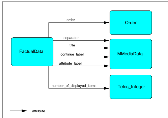
Σχήμα 3.18: Η κλάση FactualData και τα γνώρισμα που της έχουν αποδοθεί
