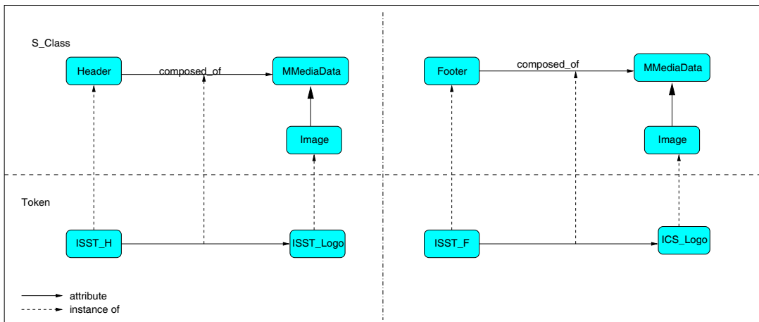
Σχήμα 3.13: Παράδειγμα Header και Footer
