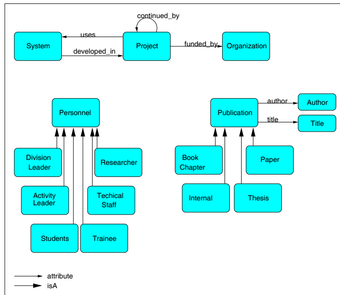
Σχήμα 3.3: Έργα, Δημοσιεύσεις και Προσωπικό
