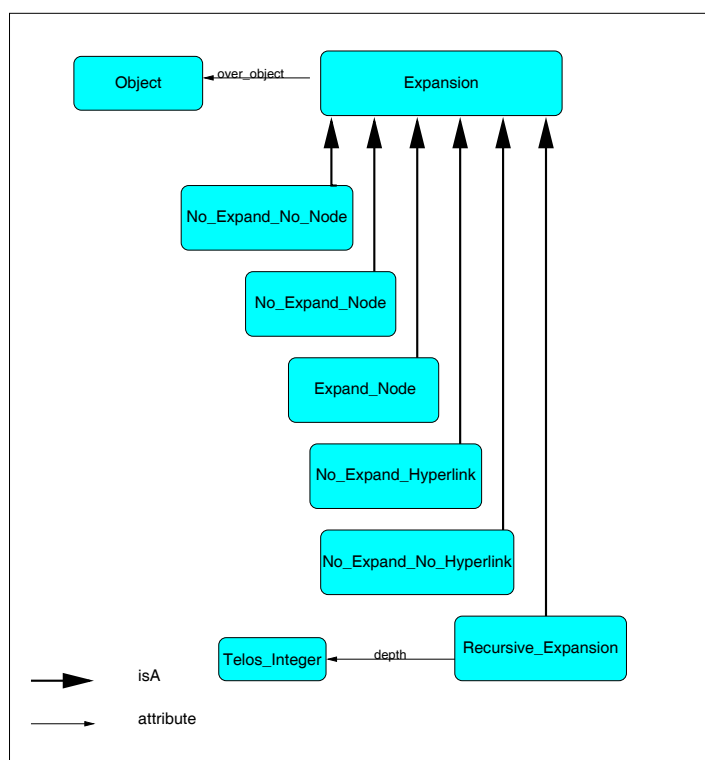
Σχήμα 3.16: Η κλάση Expansion και οι υποκλάσεις της.
