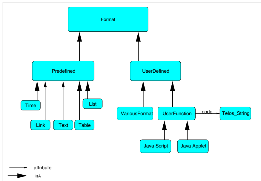
Σχήμα 3.15: Η κλάση Format και οι υποκλάσεις της.
