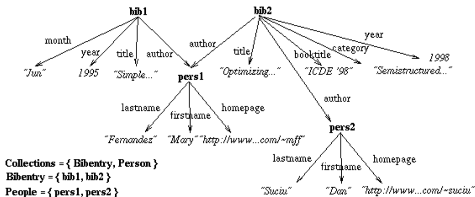
Σχήμα 2.17: Παράδειγμα γράφου δεδομένων
