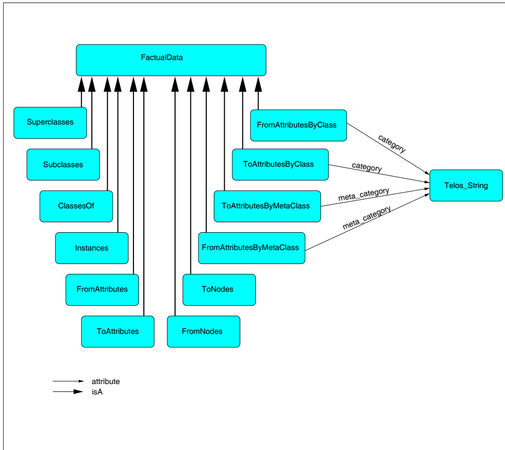
Σχήμα 3.19: Η κλάση FactualData και οι υποκλάσεις της
