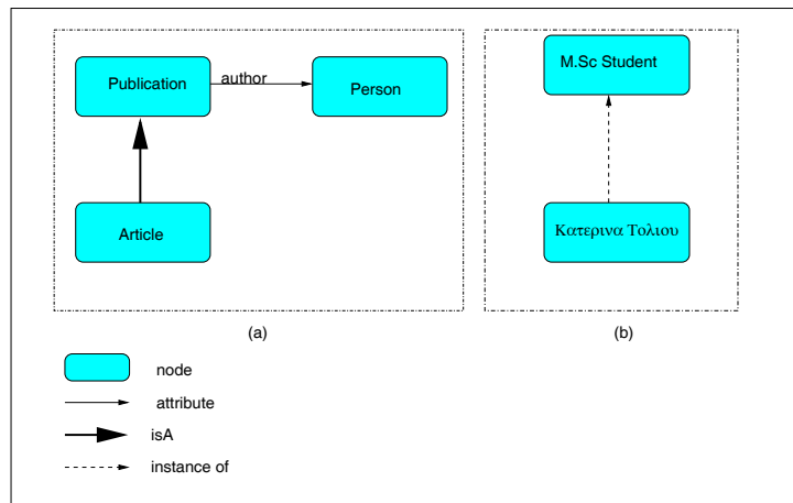
Σχήμα 3.1: Παράδειγμα κόμβων, γνωρίσματος και σχέσεων ταξινόμησης και γενίκευσης
