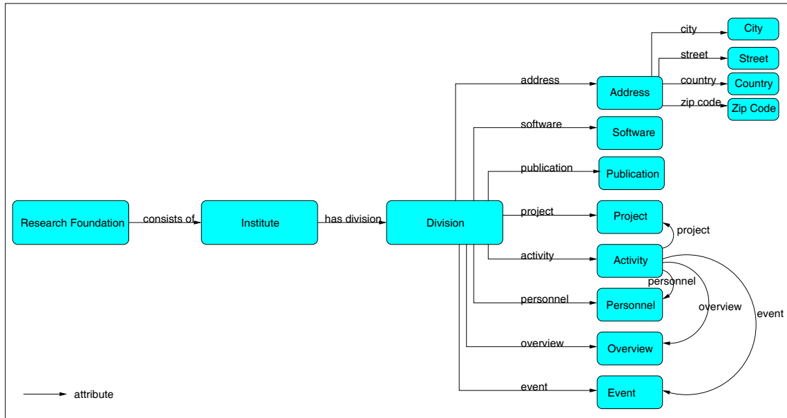
Σχήμα 3.2: Ένα Ερευνητικό Ίδρυμα αποτελείται από Ινστιτούτα και αυτά από Δραστηριότητες
