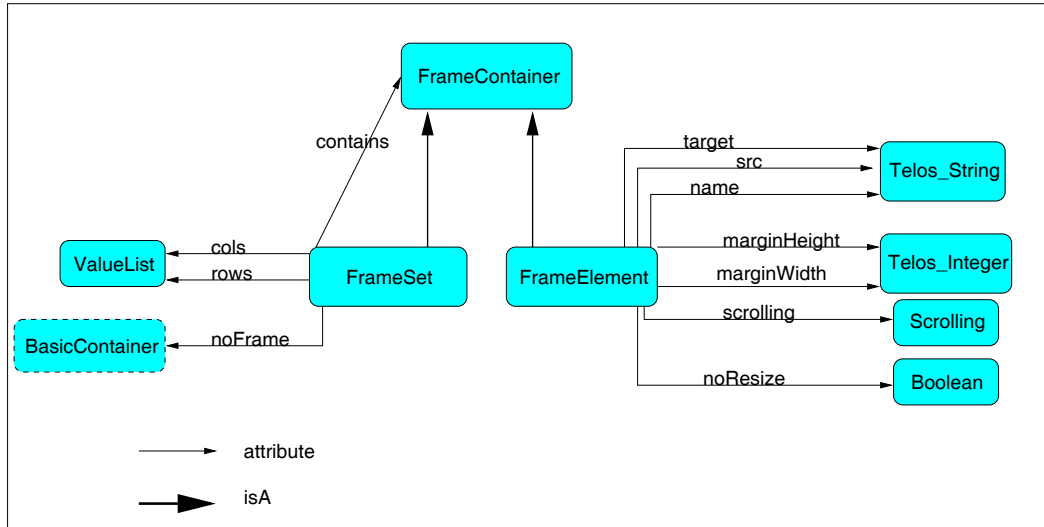
Σχήμα 3.8: Οι κλάσεις FrameContainer , FrameSet και FrameElement
