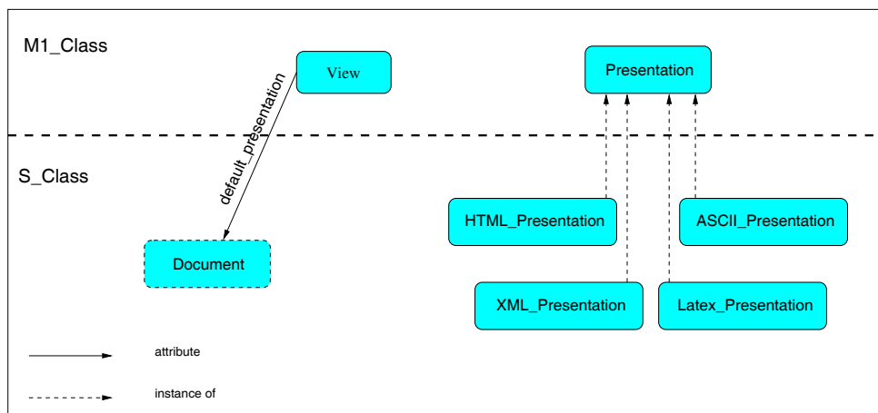
Σχήμα 3.5: Οι κλάσεις αντικειμένων View και Presentation
