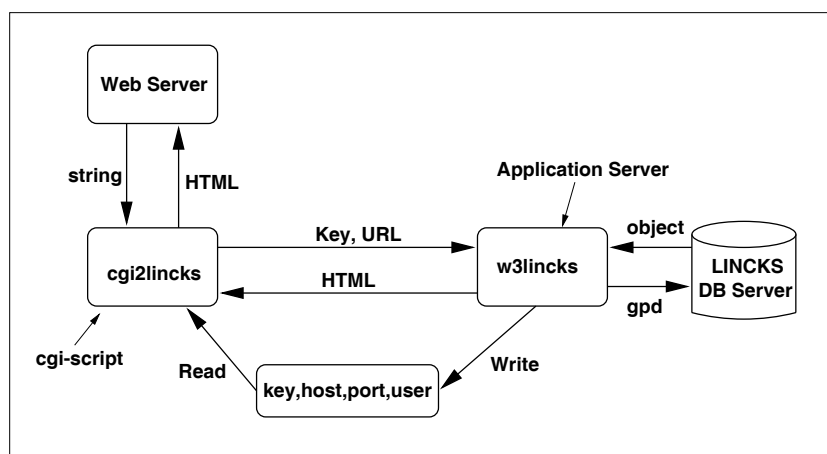
Σχήμα 2.9: Η αρχιτεκτονική που ακολουθεί το LINCKS
