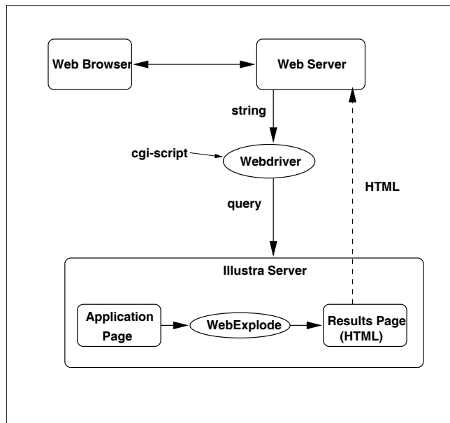
Σχήμα 2.5: Η αρχιτεκτονική που ακολουθεί το Illustra
