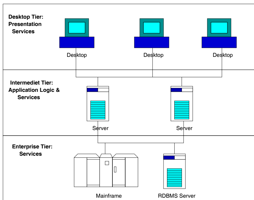
Σχήμα 2.1: Η αρχιτεκτονική τριών επιπέδων
