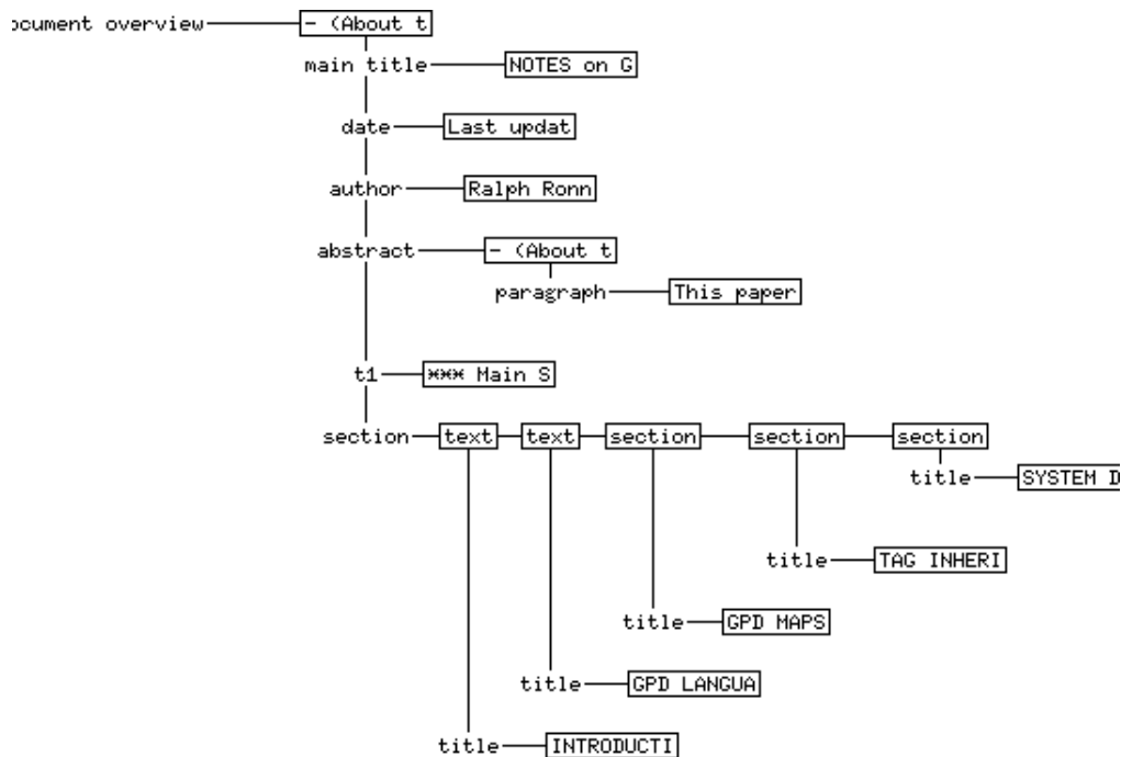
Σχήμα 2.10: Ένα παράδειγμα του τμήματος STRUCTURE ενός GPD
