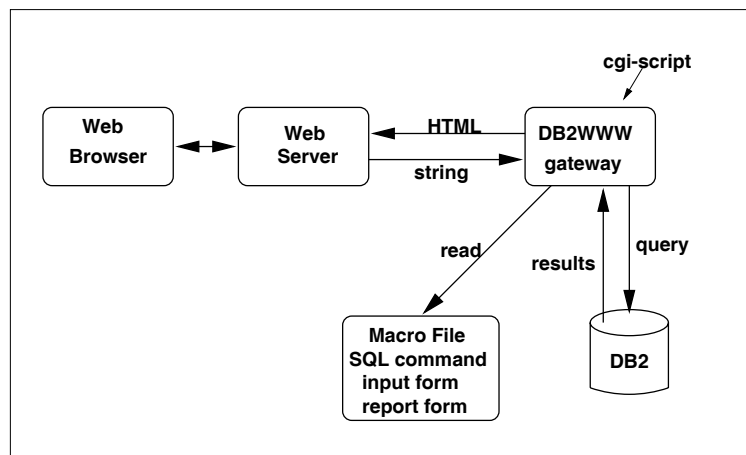
Σχήμα 2.4: Η αρχιτεκτονική που χρησιμοποιεί το DB2WWW
