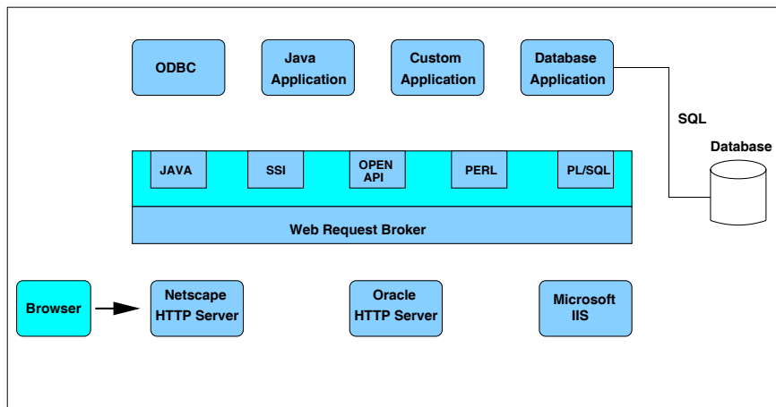
Σχήμα 2.8: Η αρχιτεκτονική που ακολουθεί η Oracle
