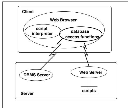
Σχήμα 2.15: Η αρχιτεκτονική Browser Extension
