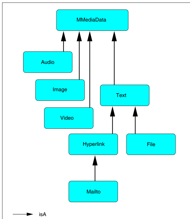
Σχήμα 3.17: Η κλάση MMediaData και οι υποκλάσεις της
