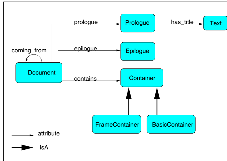
Σχήμα 3.6: Η κλάση Document και τα γνώρισματά που της έχουν αποδοθεί
