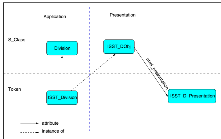
Σχήμα 3.4: Παράδειγμα προσδιορισμού παρουσίασης
