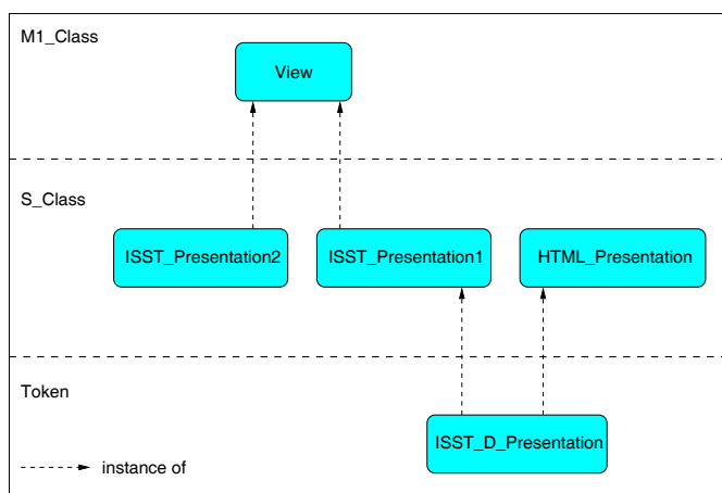
Σχήμα 3.7: Μια λογική παράσταση ταξινομείται στην όψη και το είδος διαμόρφωσης κειμένου σύμφωνα με τα οποία θα παραχθεί η παρουσίαση
