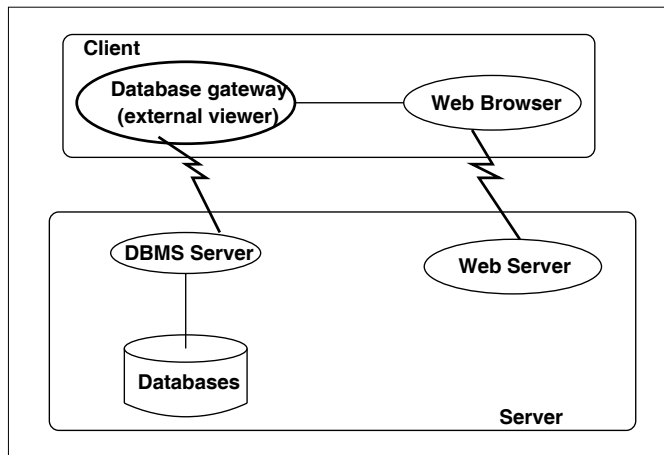
Σχήμα 2.14: Η αρχιτεκτονική External Viewer
