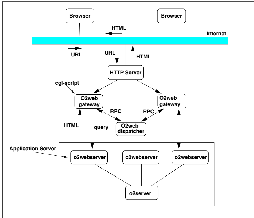
Σχήμα 2.7: Η αρχιτεκτονική που ακολουθεί η O_2 .
