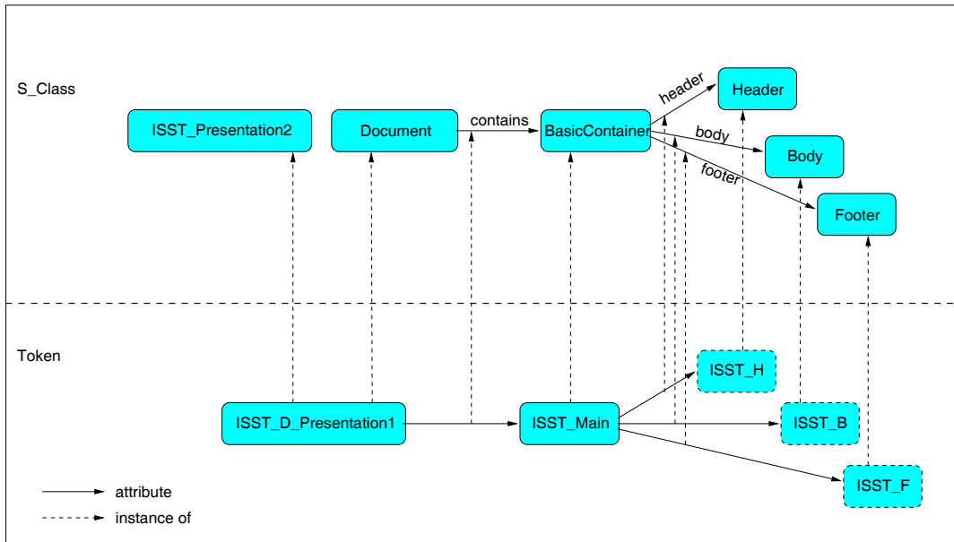
Σχήμα 3.12: Παράδειγμα χρήσης του BasicContainer
