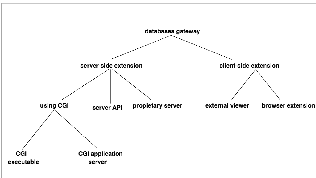
Σχήμα 2.2: Ταξινόμηση των διαφόρων αρχιτεκτονικών
