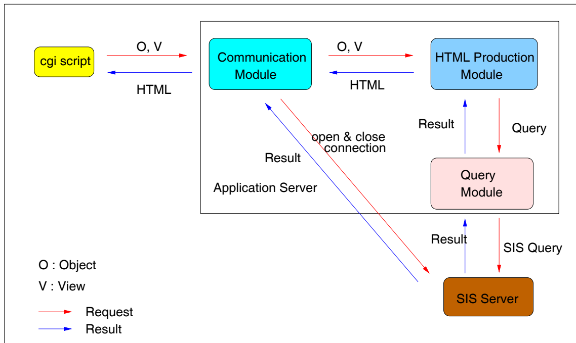
Σχήμα 4.2: Ο εξυπηρέτης εφαρμογής
