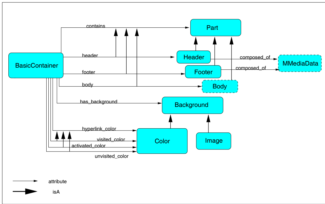
Σχήμα 3.10: Η κλάση BasicContainer και τα γνωρίσματά της.
