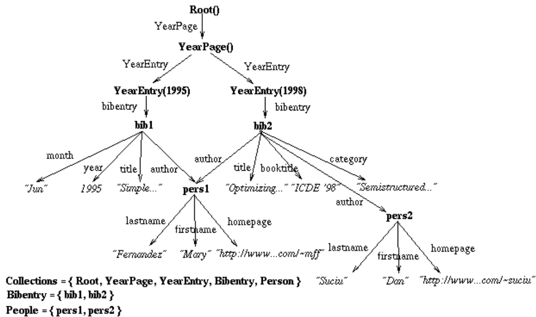
Σχήμα 2.18: Παράδειγμα γράφου ιστοκόμβων
